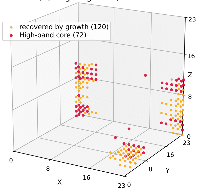
(d) Region growth, floor 20
