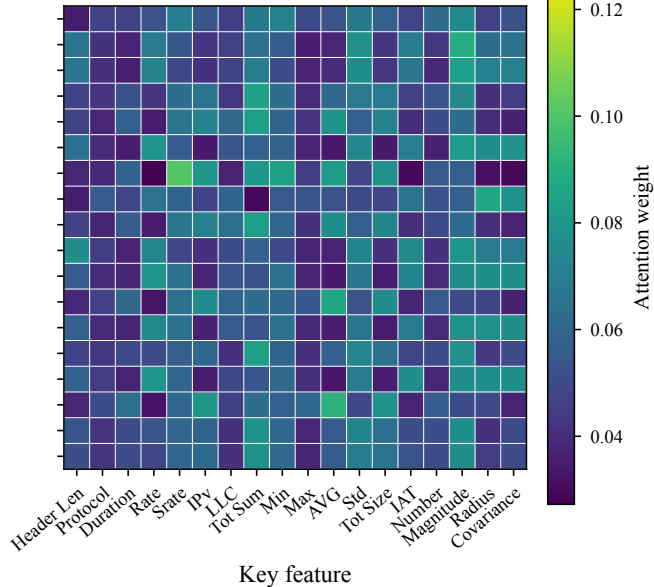
(b) Attn-Logic-KAN (no logic)
