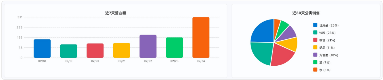
图表截图
