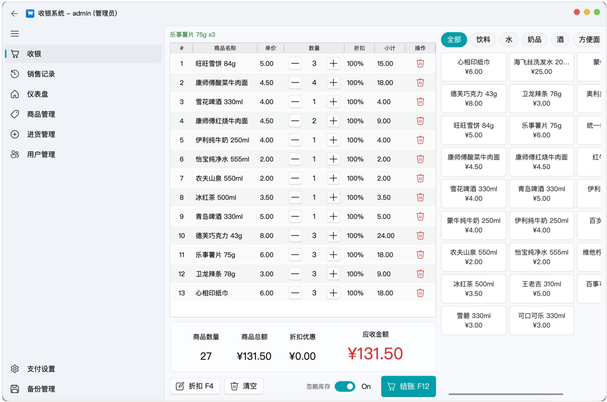
主窗口截图
