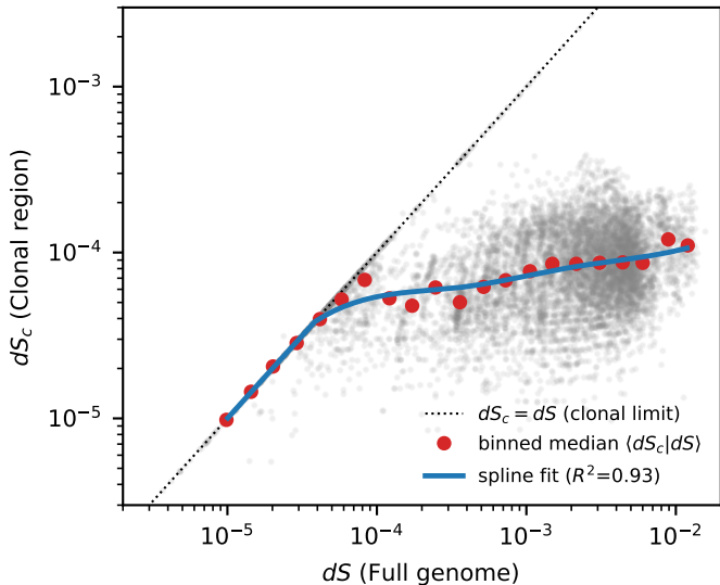
Clonal divergence accumulation \langle dS_c | dS \rangle
