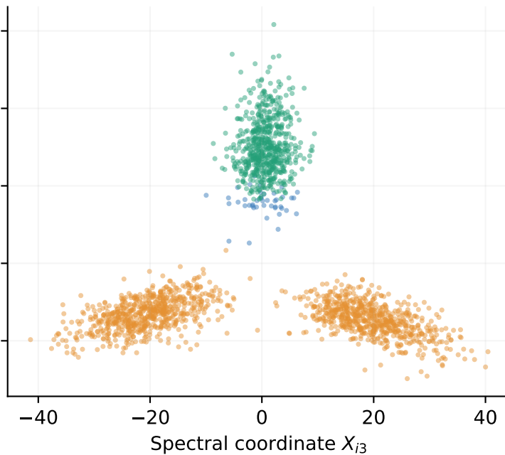
Top-subset seeds + EM 709 / 2000 errors
