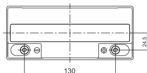
F13-BP TERMINAL
