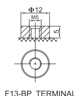
F13-BP TERMINAL
