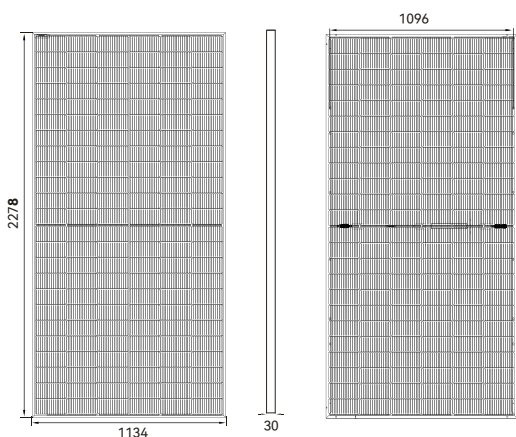
尺寸 单位: 毫米
