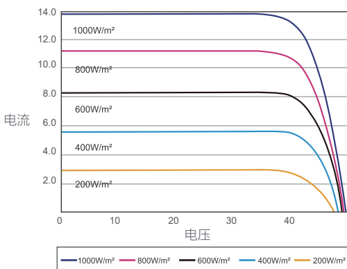
电流-电压曲线
