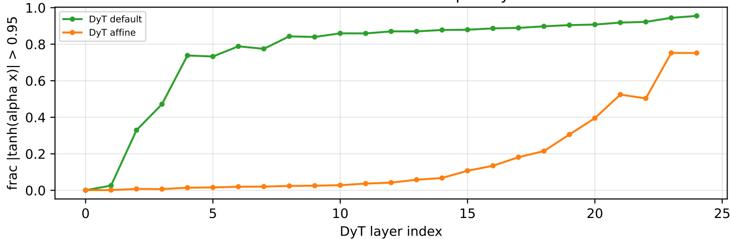
Classification: saturation per layer
