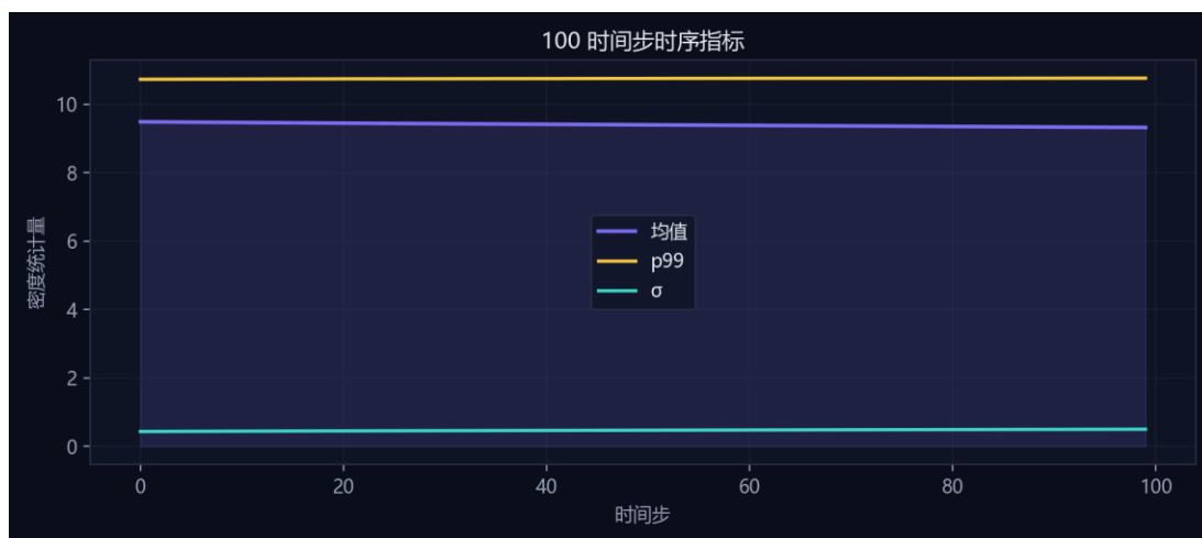
图 6 100 步 mean、p99 与 \sigma 时序曲线
