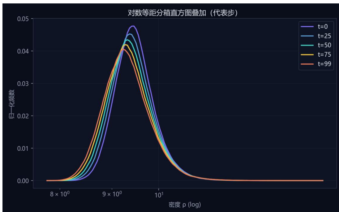
图 5 代表步 \log 直方图叠加
