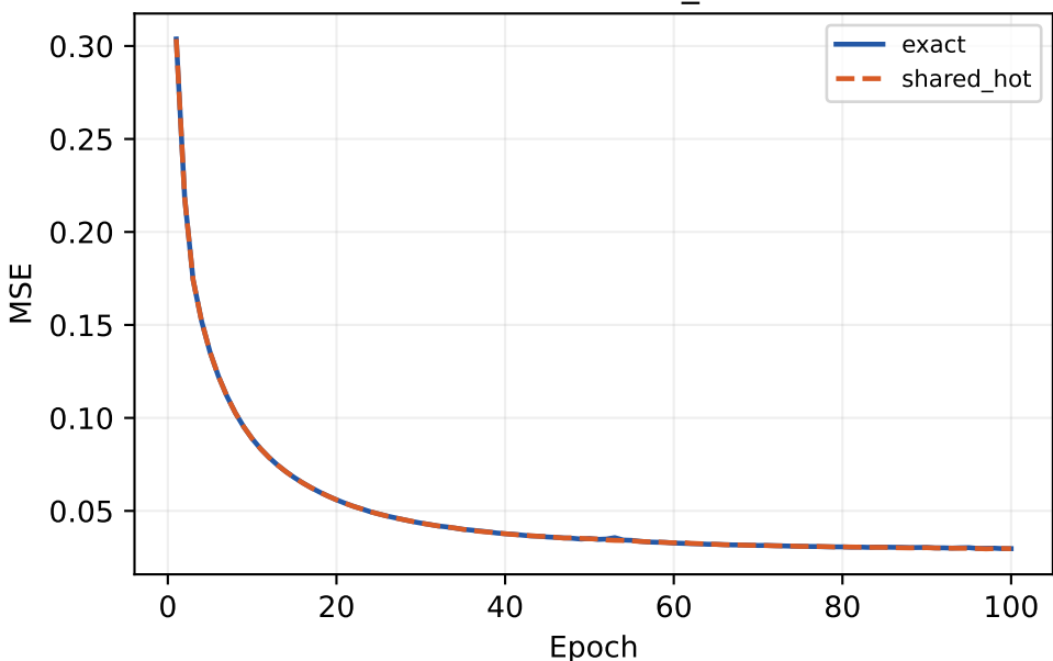
GCONV_GRU — train_mse
