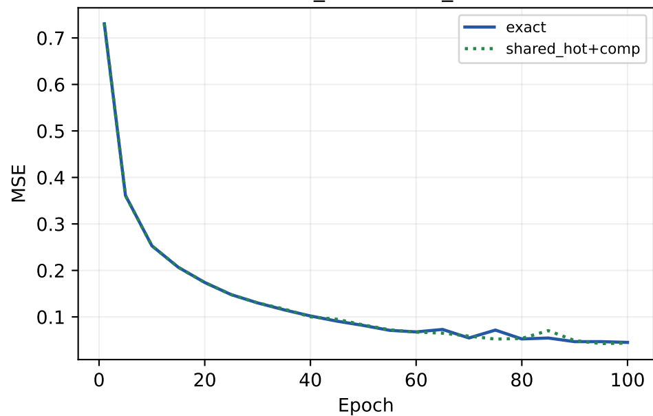
GCONV_GRU — val_mse
