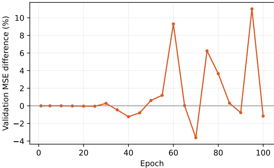
DCRNN
