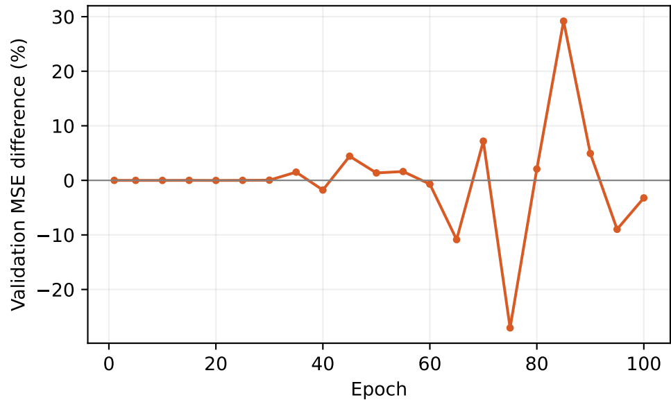
GCONV_GRU
