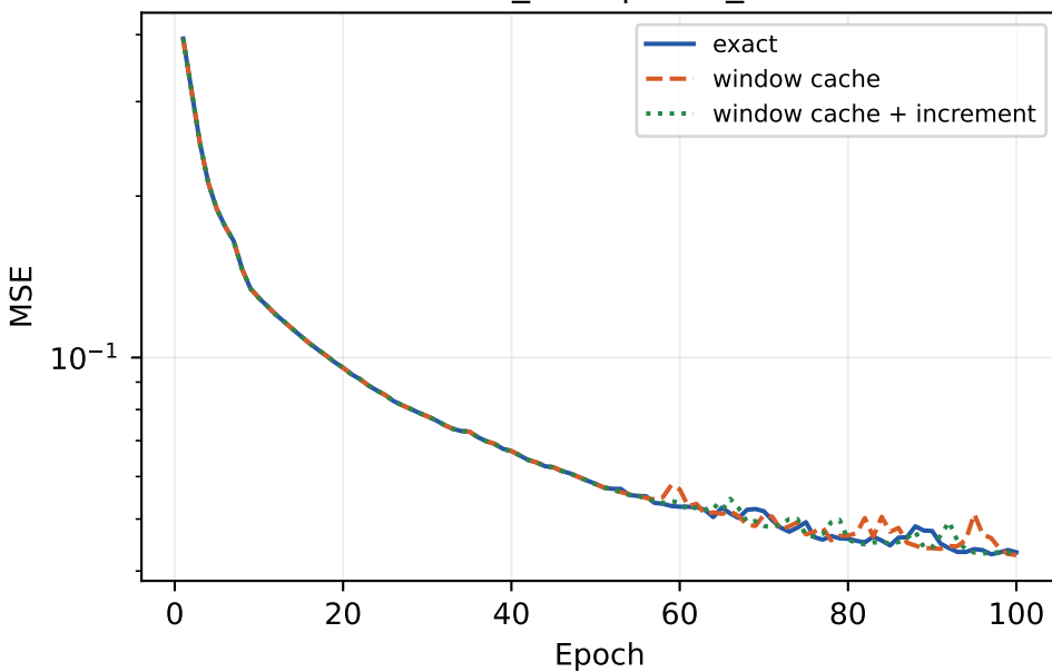
GCONV_GRU | train_mse
