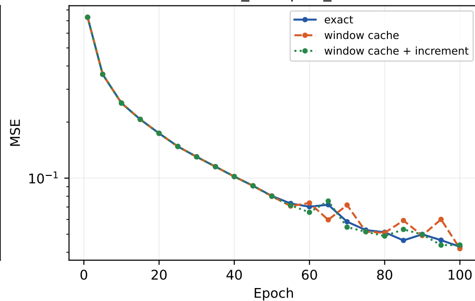
GCONV_GRU | val_mse
