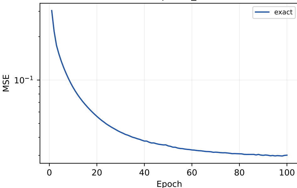
GCONV_GRU | train_mse
