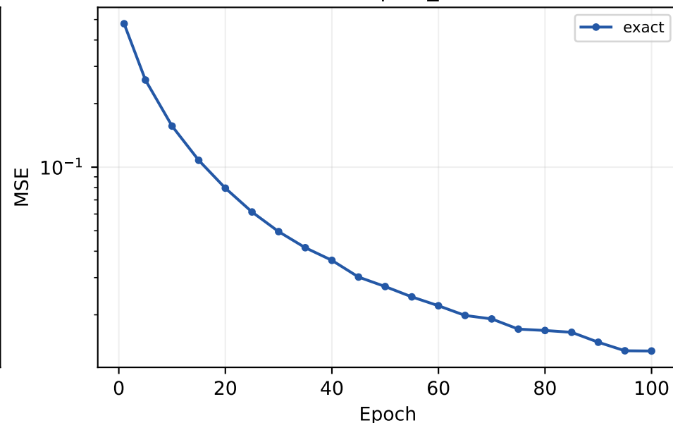
GCONV_GRU | val_mse
