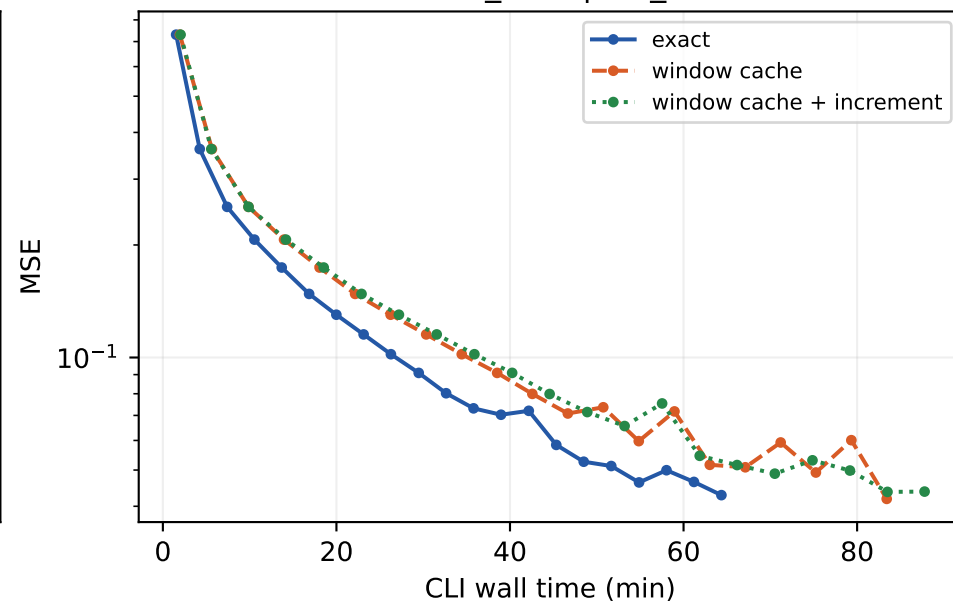
GCONV_GRU | val_mse
