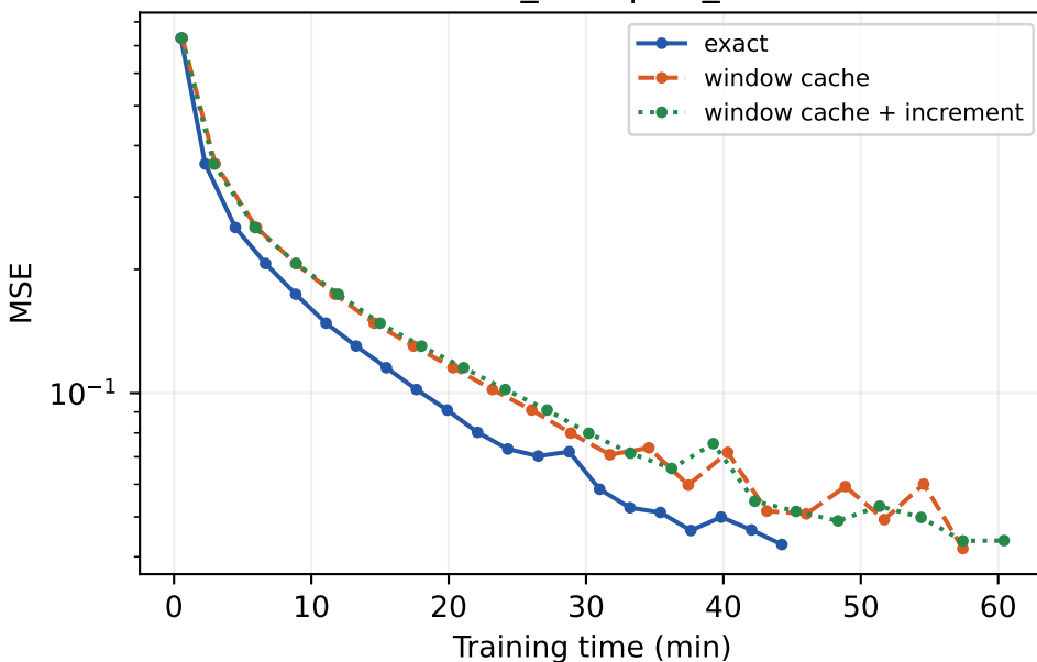
GCONV_GRU | val_mse
