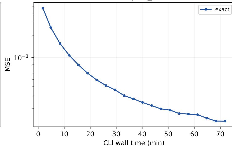
GCONV_GRU | val_mse
