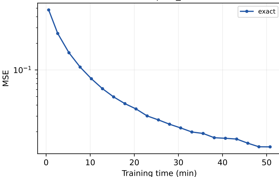
GCONV_GRU | val_mse
