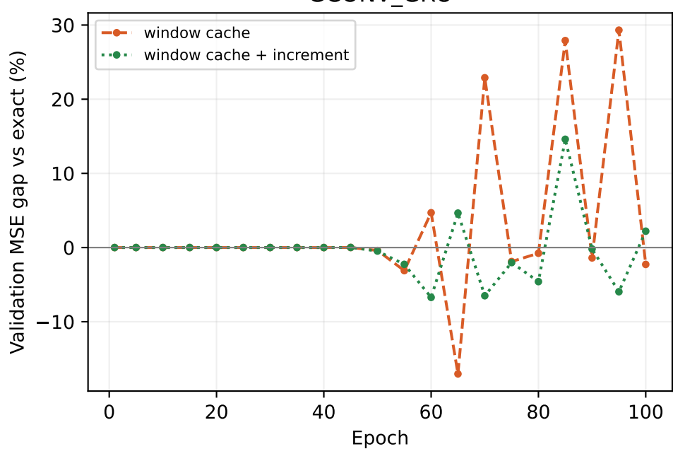
GCONV_GRU
