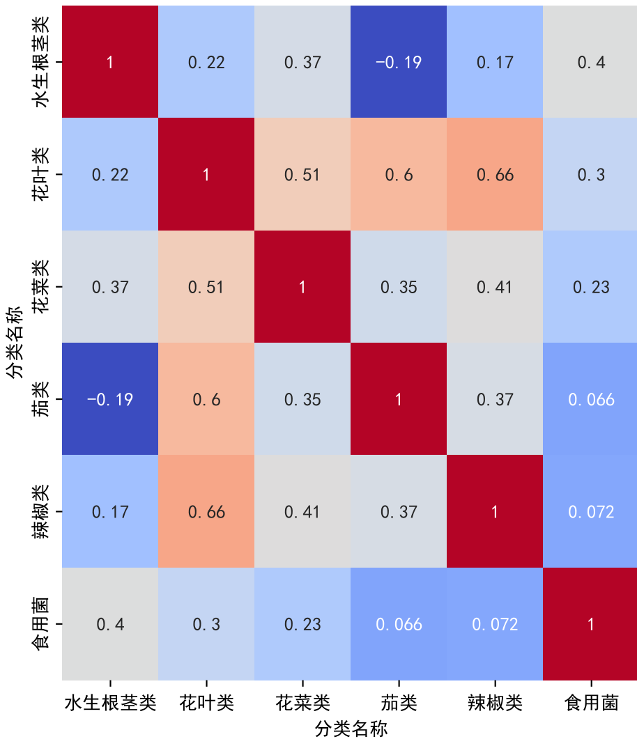
皮尔逊相关系数
