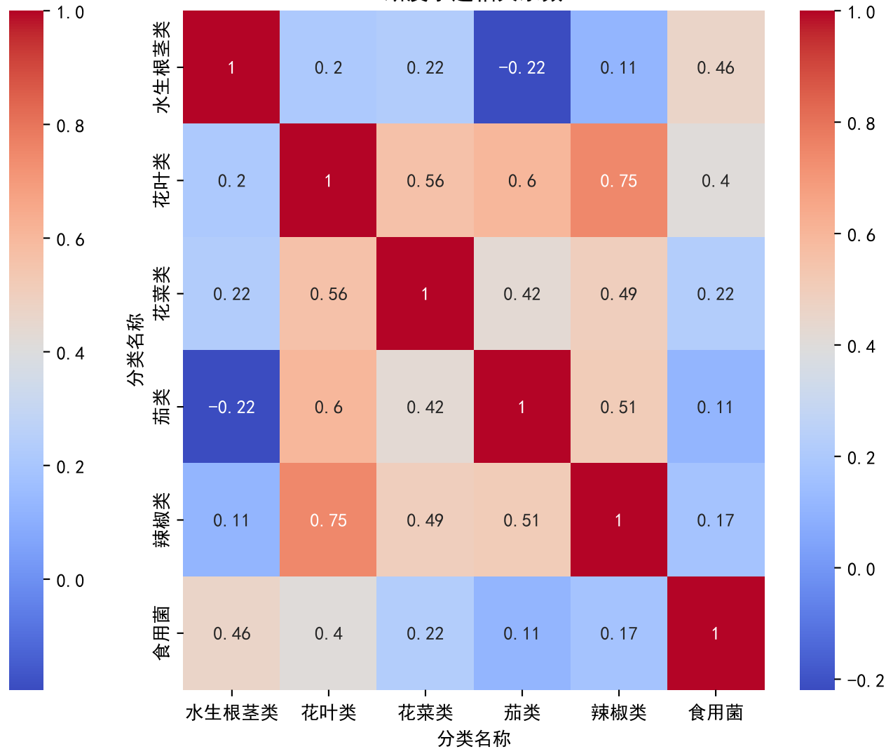
两种相关系数热力图
