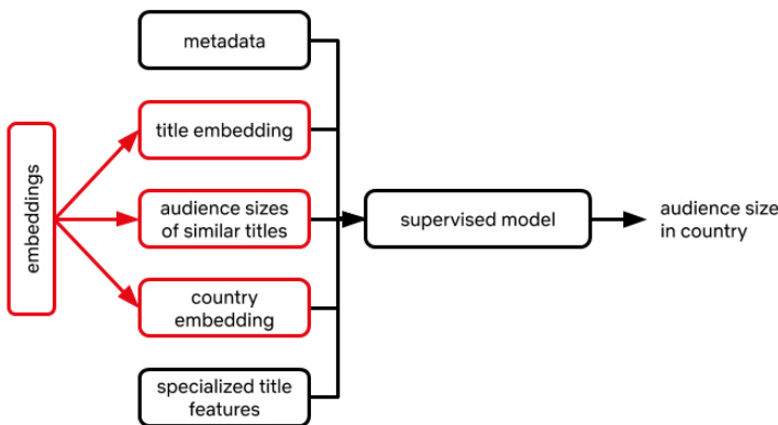
[그림 3-9] 시청자 규모 예측을 위한 전이학습 모델
