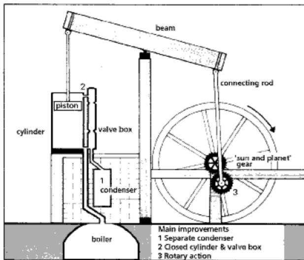
[그림 7-2] 와트의 증기기관 - 기계 동력 생산의 확산
