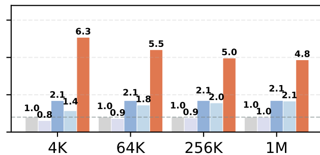
Llama4-Maverick, BS=4
