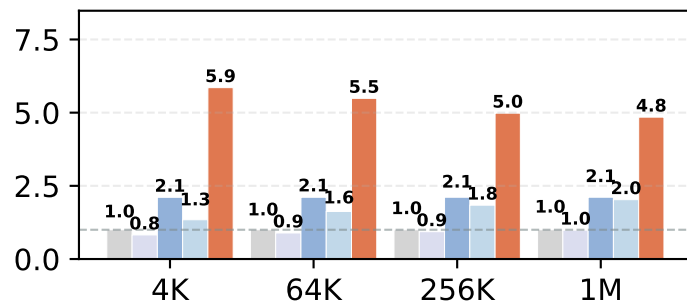
Llama4-Maverick, BS=1
