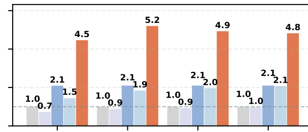
Qwen3-235B, BS=16
