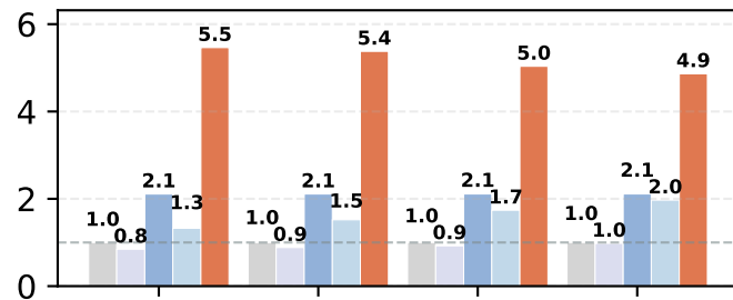
Qwen3-235B, BS=1
