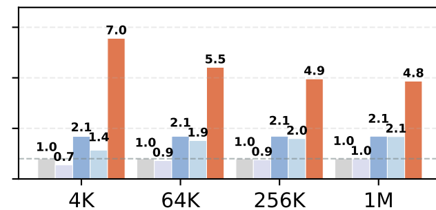
Llama4-Maverick, BS=32
