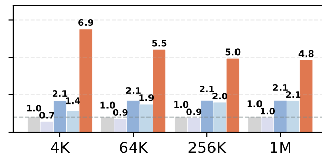
Llama4-Maverick, BS=16
