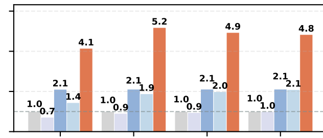
Qwen3-235B, BS=32
