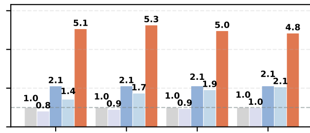
Qwen3-235B, BS=4
