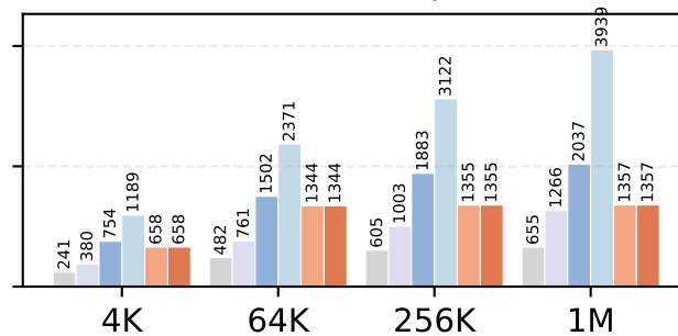
Llama4-Maverick, BS=16
