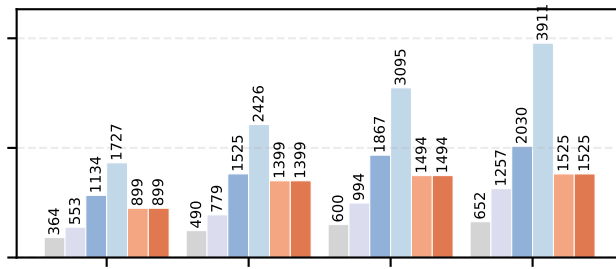
Qwen3-235B, BS=4
