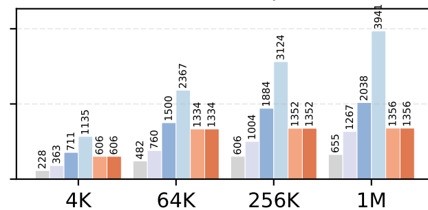
Llama4-Maverick, BS=32
