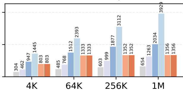
Llama4-Maverick, BS=4
