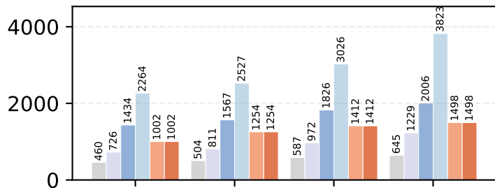
Qwen3-235B, BS=1
