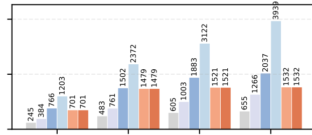
Qwen3-235B, BS=32
