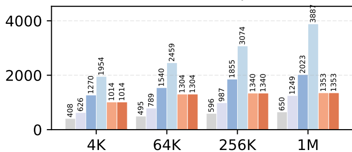
Llama4-Maverick, BS=1
