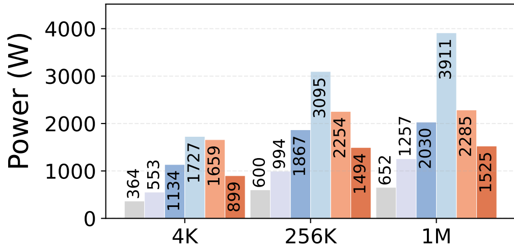
Qwen3-235B, BS=4
