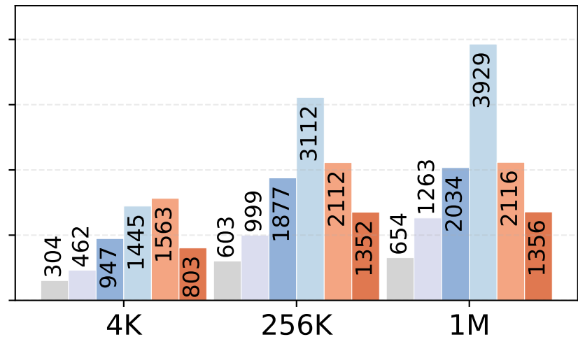
Llama4-Maverick, BS=4
