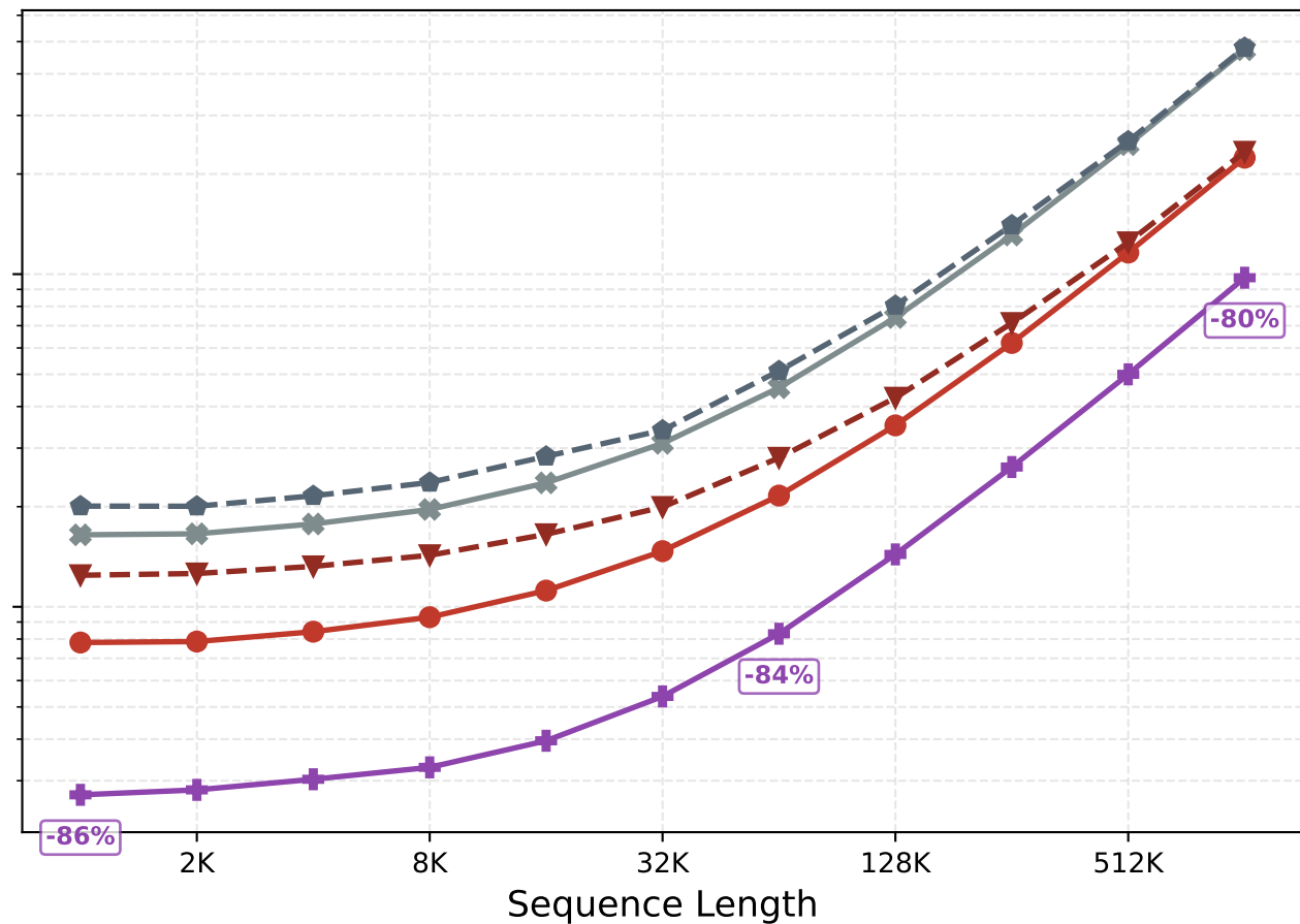
Llama4-Maverick
