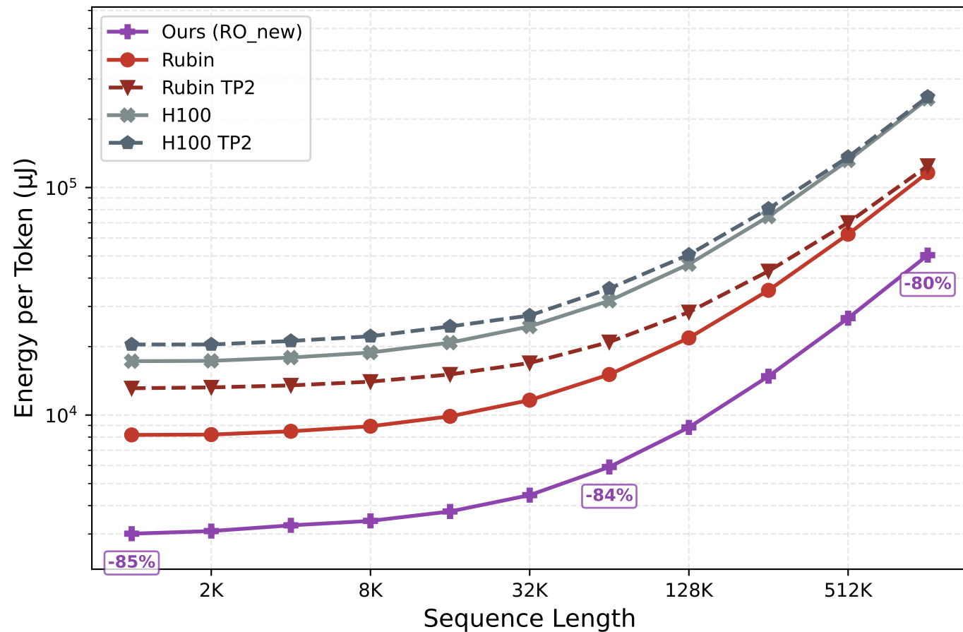
Qwen3-235B
