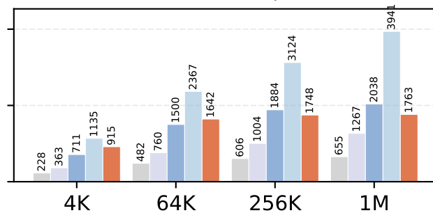
Llama4-Maverick, BS=32
