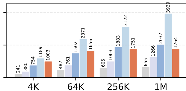
Llama4-Maverick, BS=16
