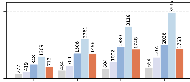
Qwen3-235B, BS=16
