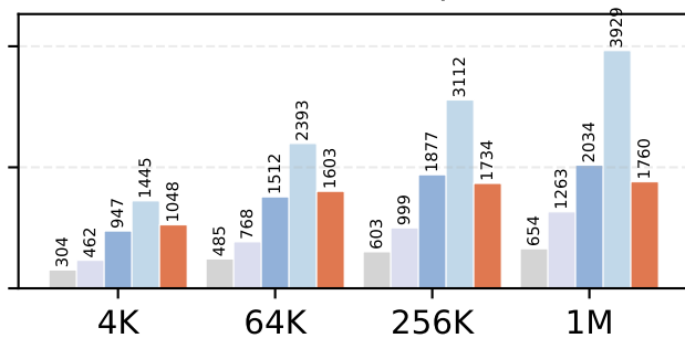
Llama4-Maverick, BS=4
