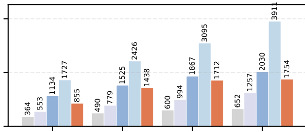
Qwen3-235B, BS=4
