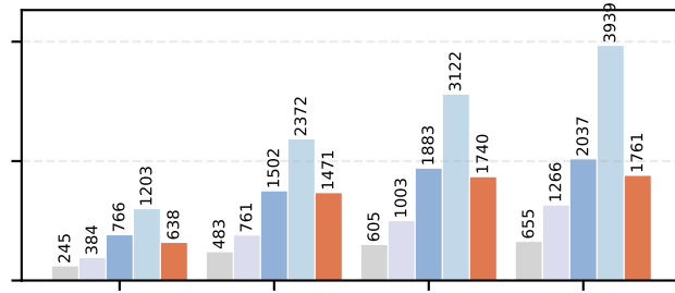
Qwen3-235B, BS=32
