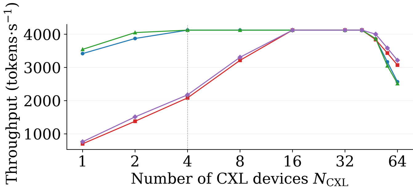
(a) Llama2-13B (MHA)
