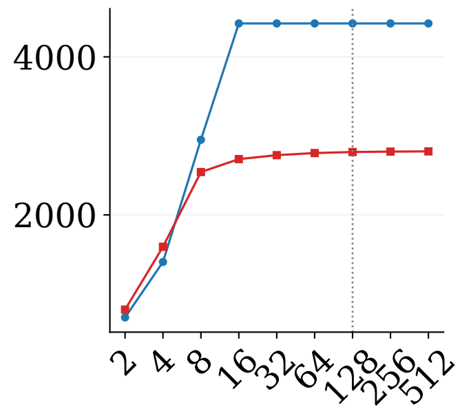
(b) CXL link BW (GB/s)
