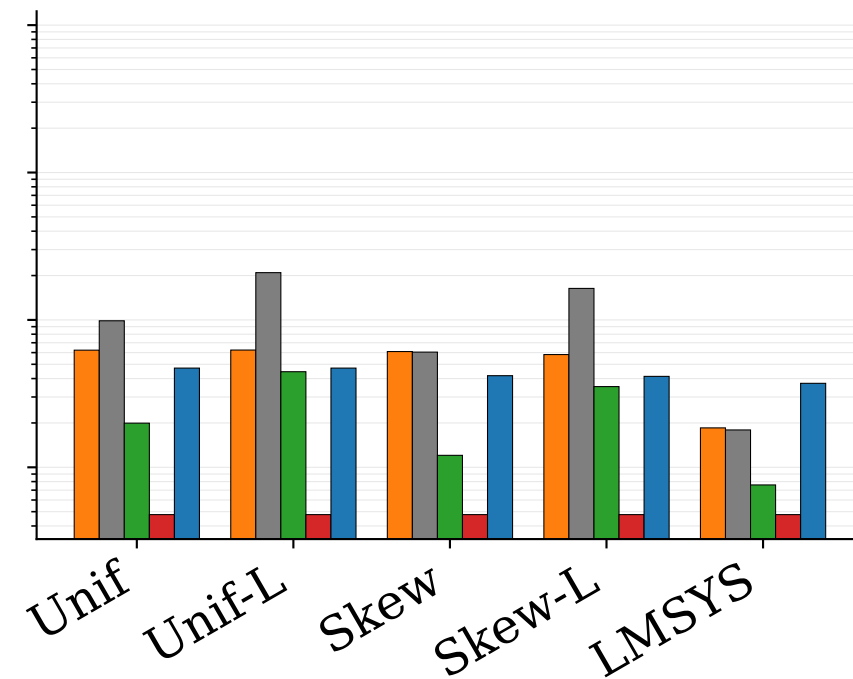
(c) Llama3-8B (GQA)
