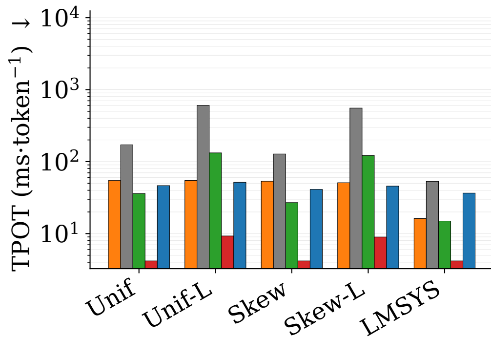
(a) Llama2-7B (MHA)
