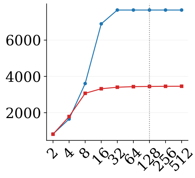
(b) CXL link BW (GB/s)
