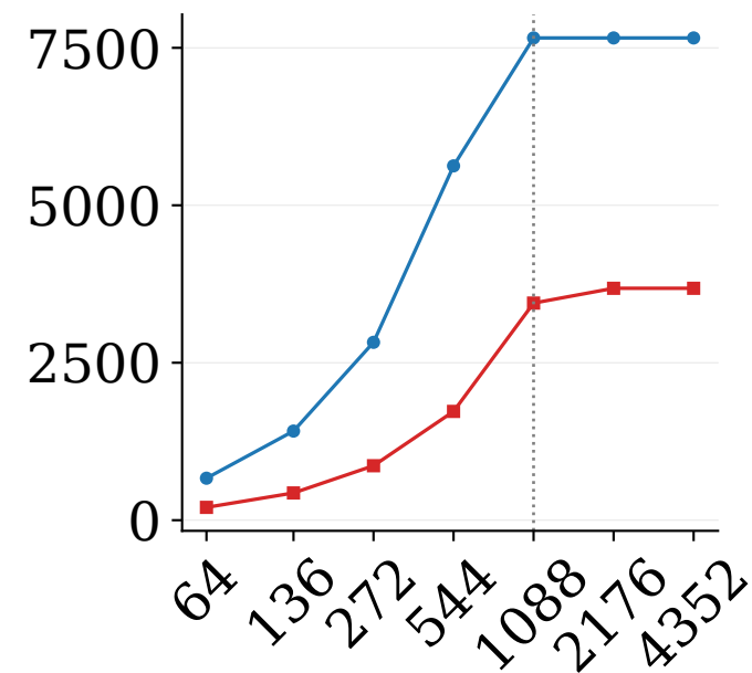
(d) Device DRAM BW (GB/s)
