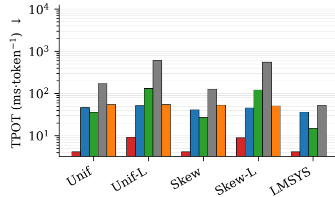
(a) Llama2-7B (MHA)
