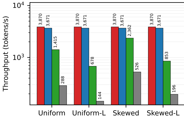
(a) Llama3-8B
