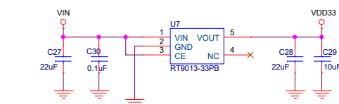
3.3V电源模块
