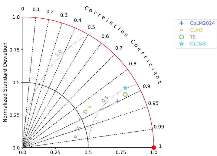
图 9: 潜热 Taylor 图（四模式对 ILAMB-FLUXCOM）。
