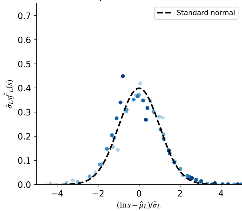
(d) Empirical standardization
