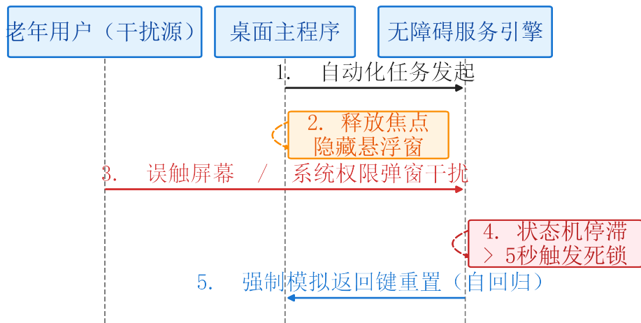
图 2.5 面临用户误触与弹窗干扰时的焦点退避与心跳防死锁时序图
