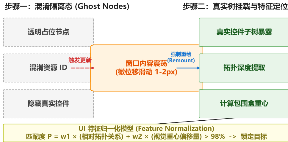
图 2.4 基于窗口内容震荡与层级拓扑指纹的主动探测机制原理图
