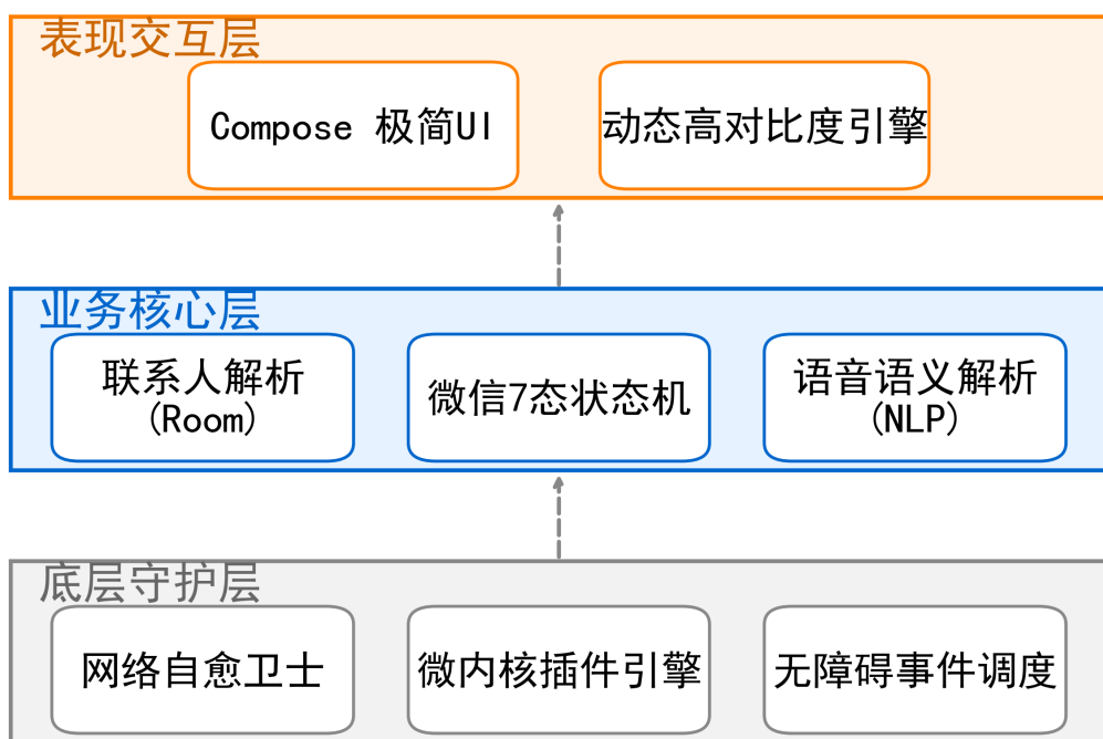
图 1.4 SimpleDesktop 系统技术全景架构图
