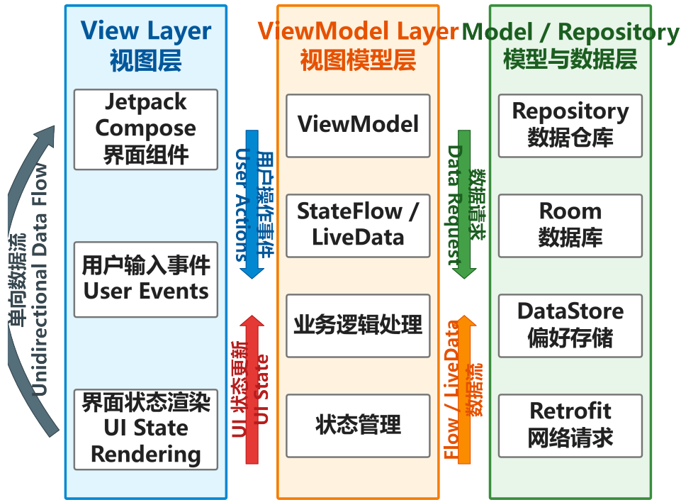
图 2.1 MVVM 架构与单向数据流工作机制
