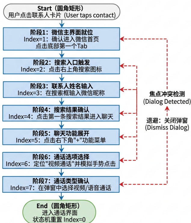
图 3.4 微信一键直拨七阶段状态机流程
