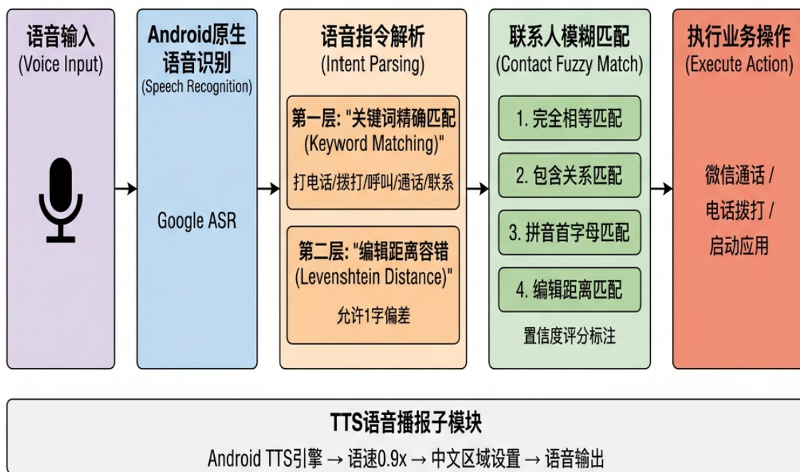
图 3.6 语音辅助模块工作流程
