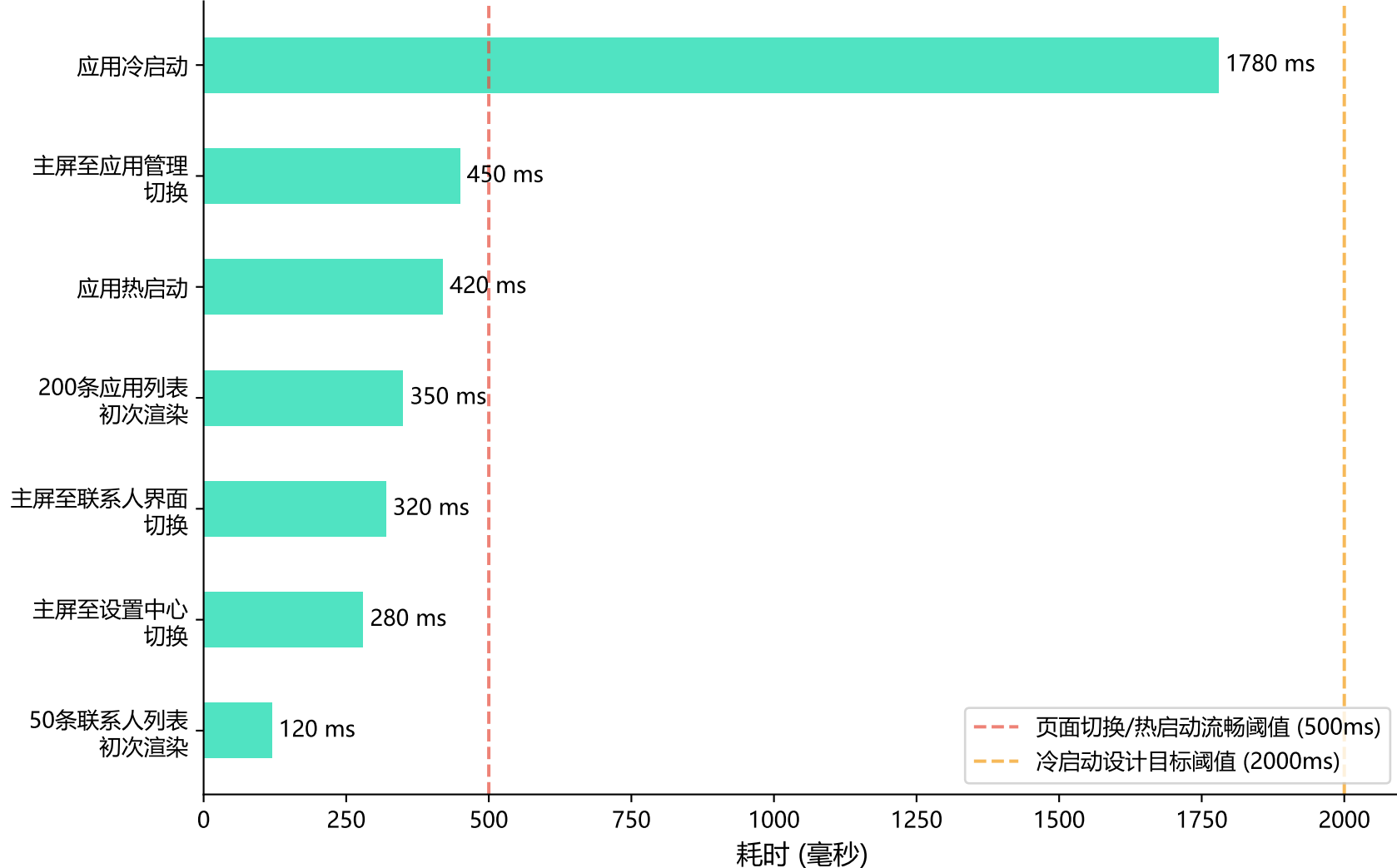
关键场景页面加载与切换速度测试结果
