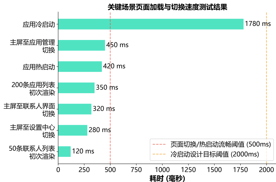
图 4.5 关键场景页面加载与切换耗时统计
