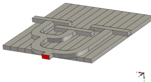
(b) 馈电层模型
