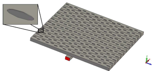
(a) 辐射体结构模型
