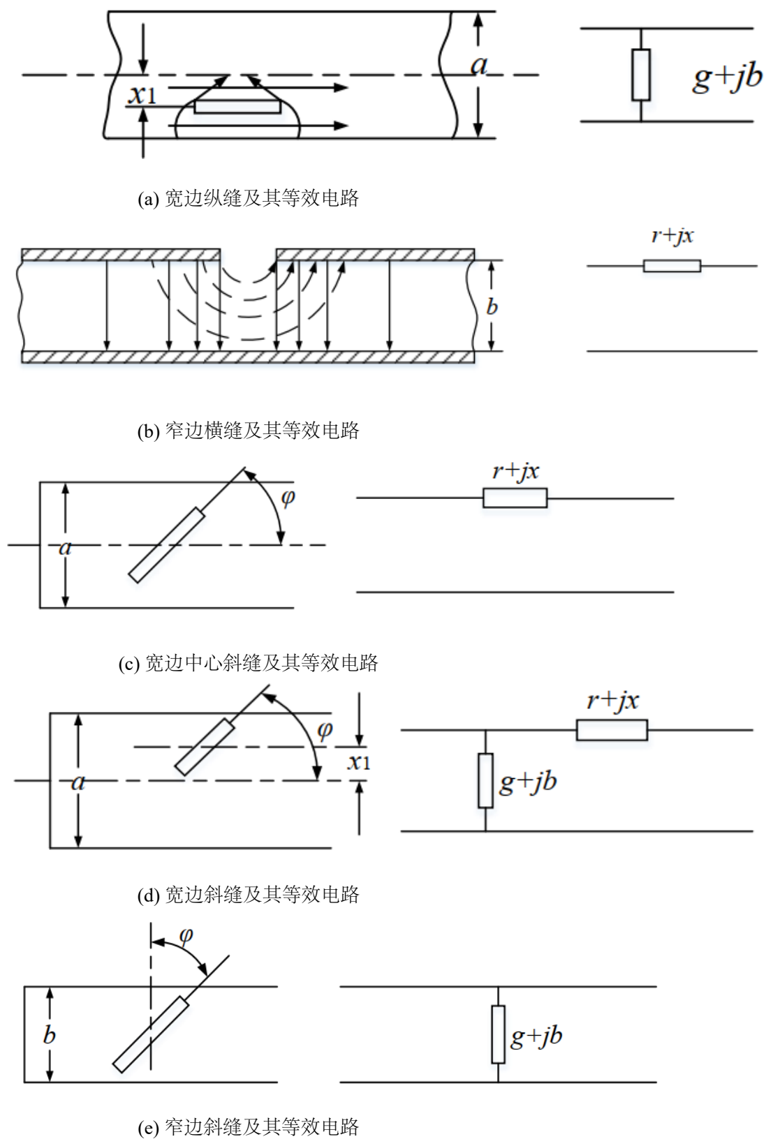
图 2.5 波导缝隙形式及其等效电路示意图
