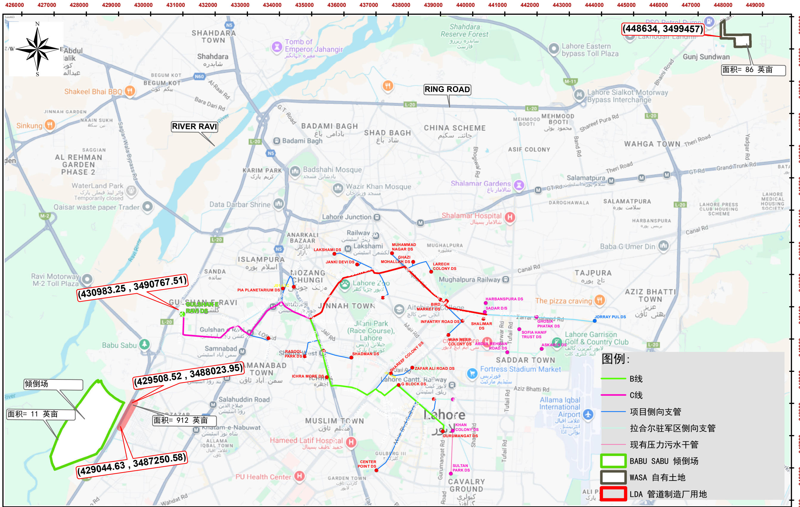
拉合尔废水与排水管理项目（LWDMP）- 从 LARECHS COLONY 到 GULSHAN-E-RAVI 的污水系统（采用非开挖技术）
