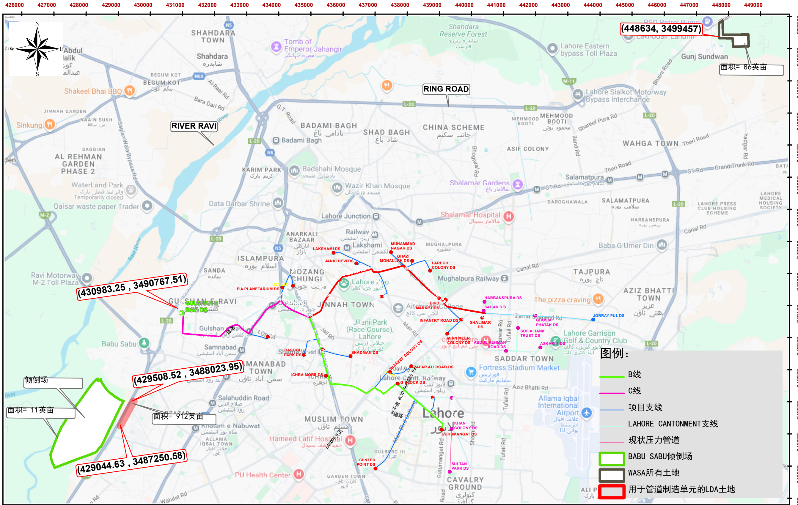
LAHORE废水与排水管理项目（LWDMP）- 从LARECHS COLONY至GULSHAN-E-RAVI、LAHORE的排水系统（采用非开挖技术）
