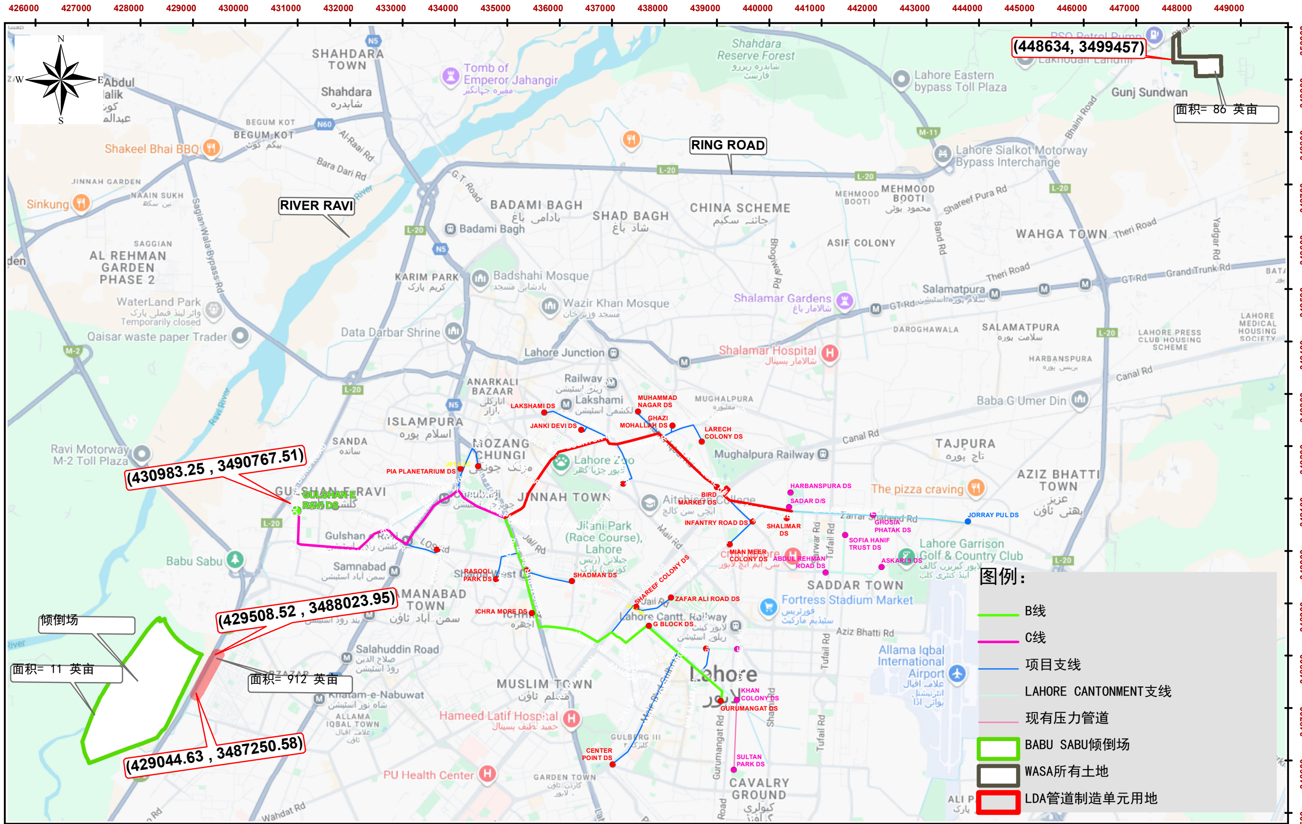
LAHORE污水和排水管理项目（LWDMP）- 从LARECHS COLONY至GULSHAN-E-RAVI、LAHORE的污水管网（采用非开挖技术）
