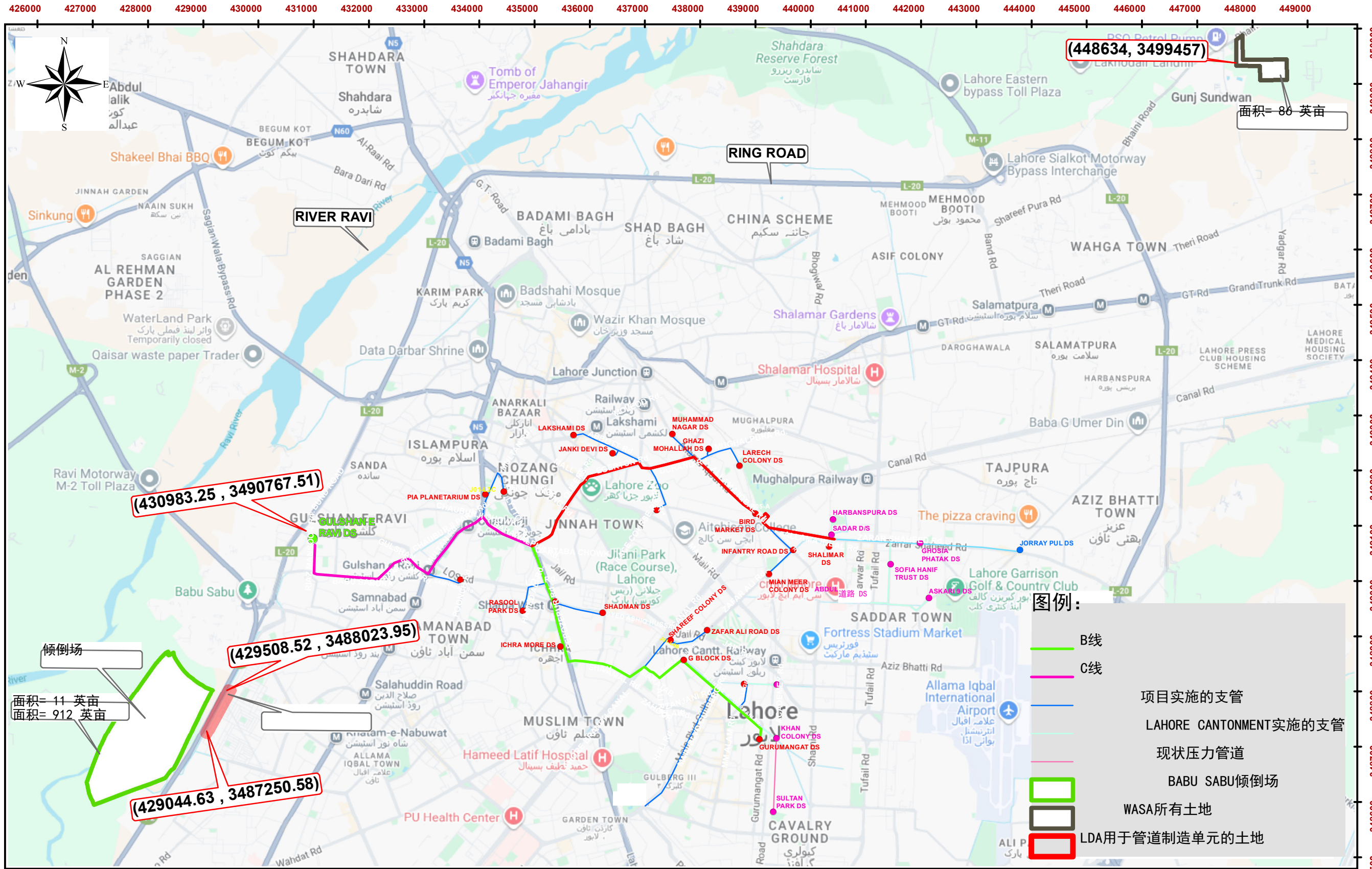
LAHORE污水和排水管理项目（LWDMP）- 从LARECHS COLONY至GULSHAN-E-RAVI、LAHORE的污水管道系统（采用非开挖技术）
