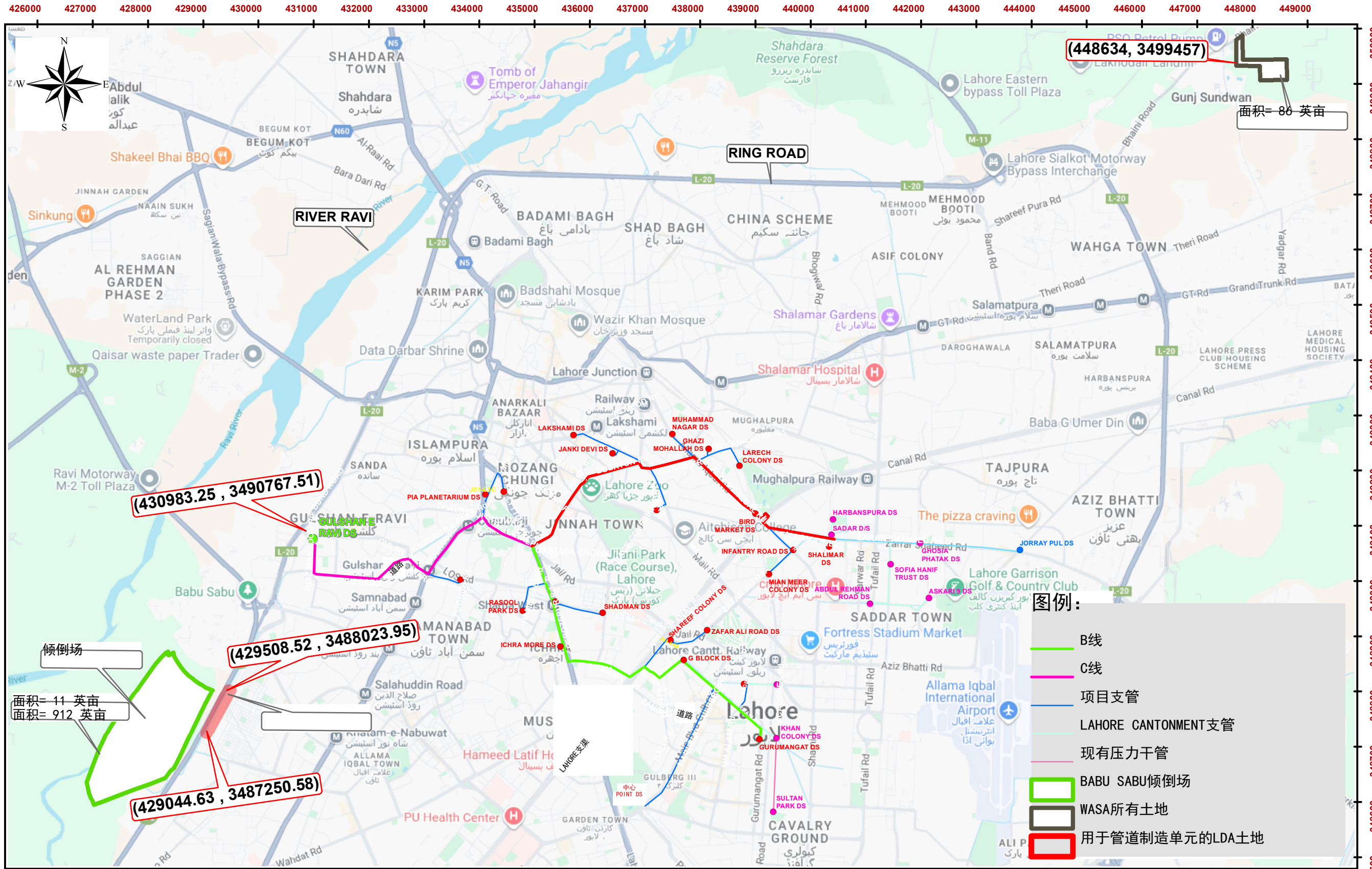
LAHORE废水与排水管理项目（LWDMP）- LARECHS COLONY至GULSHAN-E-RAVI的污水管网，LAHORE（采用非开挖技术）
