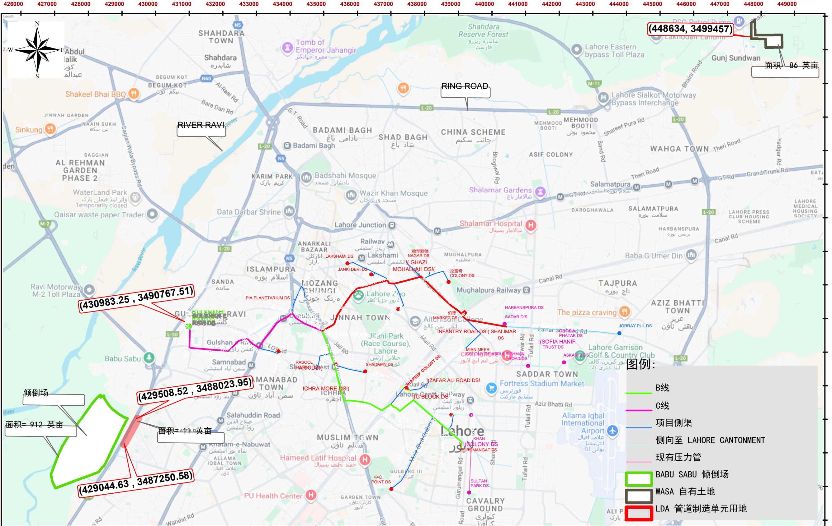
拉合尔废水与排水管理项目（LWDMP）- 从 LARECHS COLONY 到 GULSHAN-E-RAVI, LAHORE 的污水系统（采用非开挖技术）
