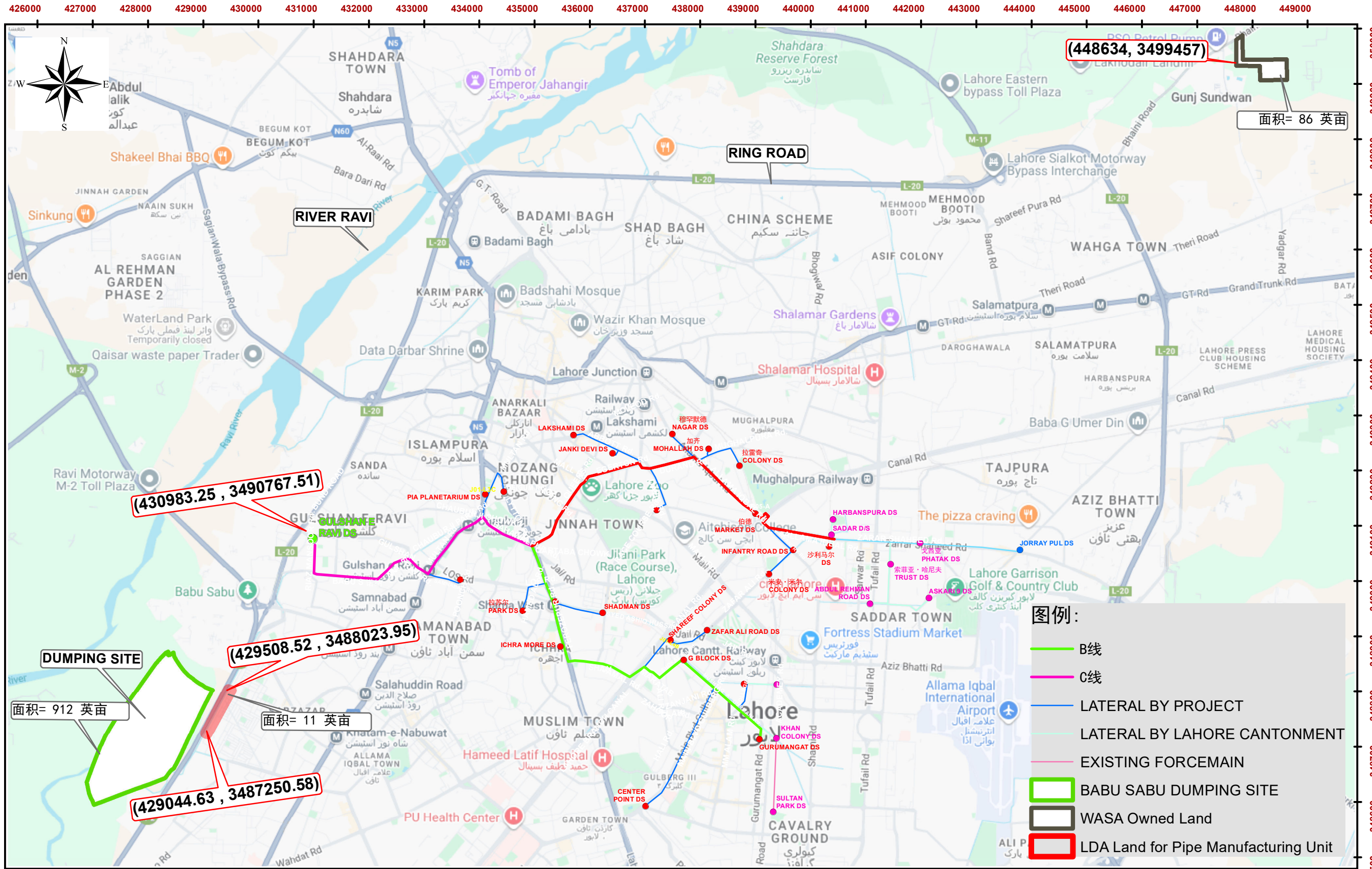
拉合尔废水与排水管理项目 (LWDMP) - 从 LARECHS COLONY 到 GULSHAN-E-RAVI 的污水系统, 拉合尔 (采用非开挖技术)
