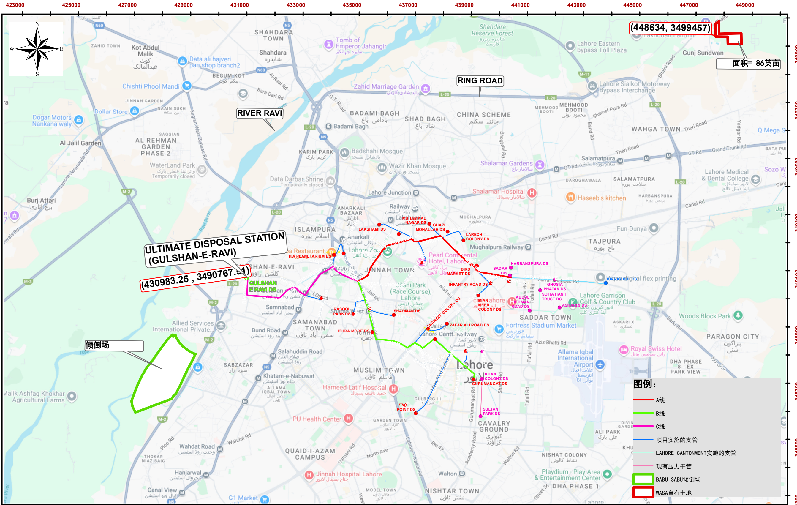
拉合尔污水与排水管理项目（LWDMP）——从LARECHS COLONY至GULSHAN-E-RAVI的污水系统，拉合尔（采用非开挖技术）
