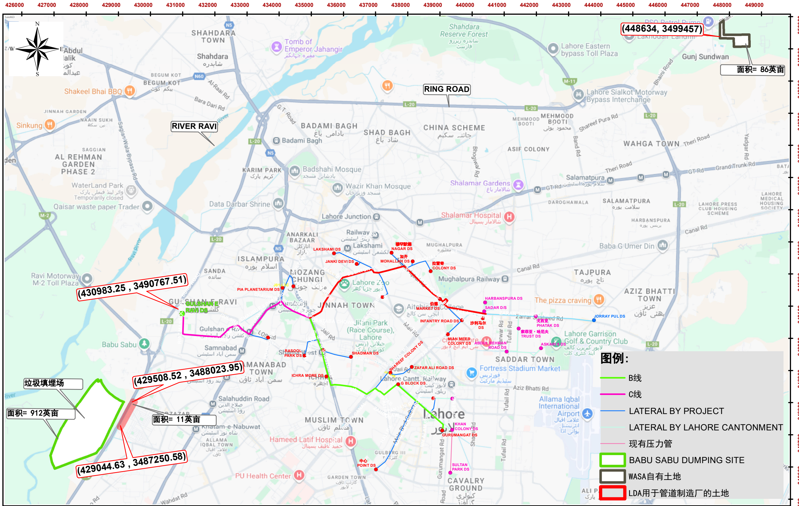
拉合尔废水与排水管理项目 (LWDMP) - 从LARECHS COLONY到GULSHAN-E-AVI的污水系统，拉合尔（采用非开挖技术）
