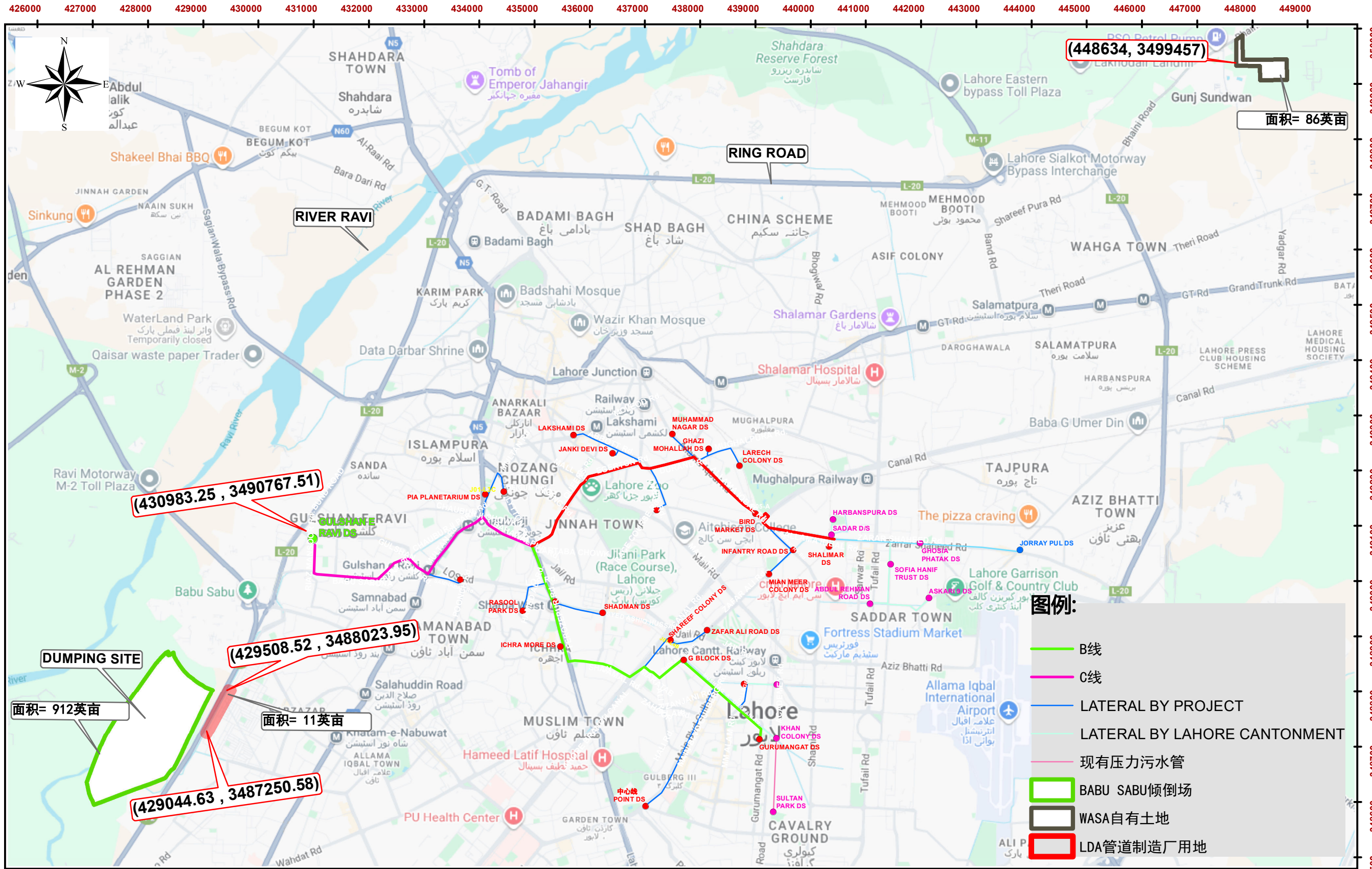
拉合尔废水与排水管理项目 (LWDMP) - 从LARECHS COLONY至GULSHAN-E-RAVI的下水道系统, LAHORE (采用非开挖技术)
