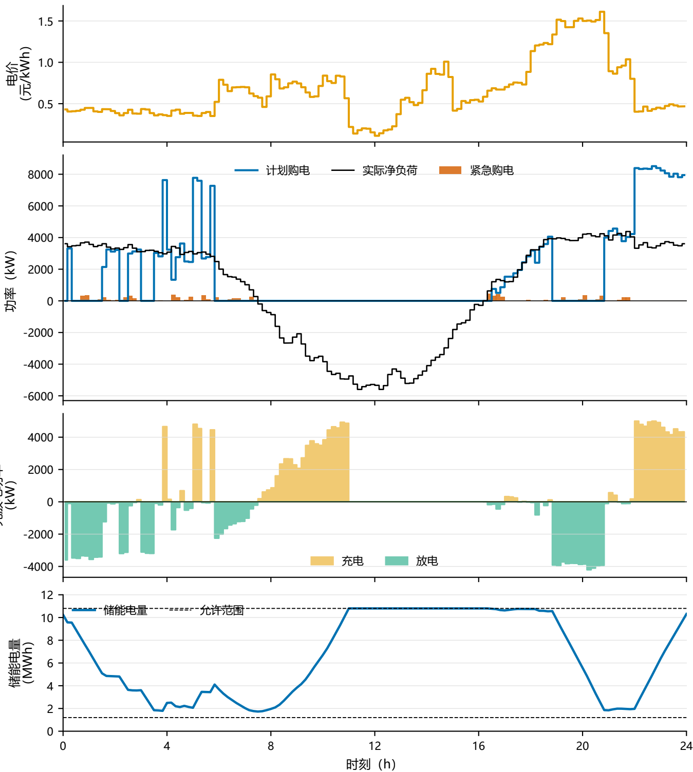
动态电价下的购电—储能协同响应 (2025-08-15)
