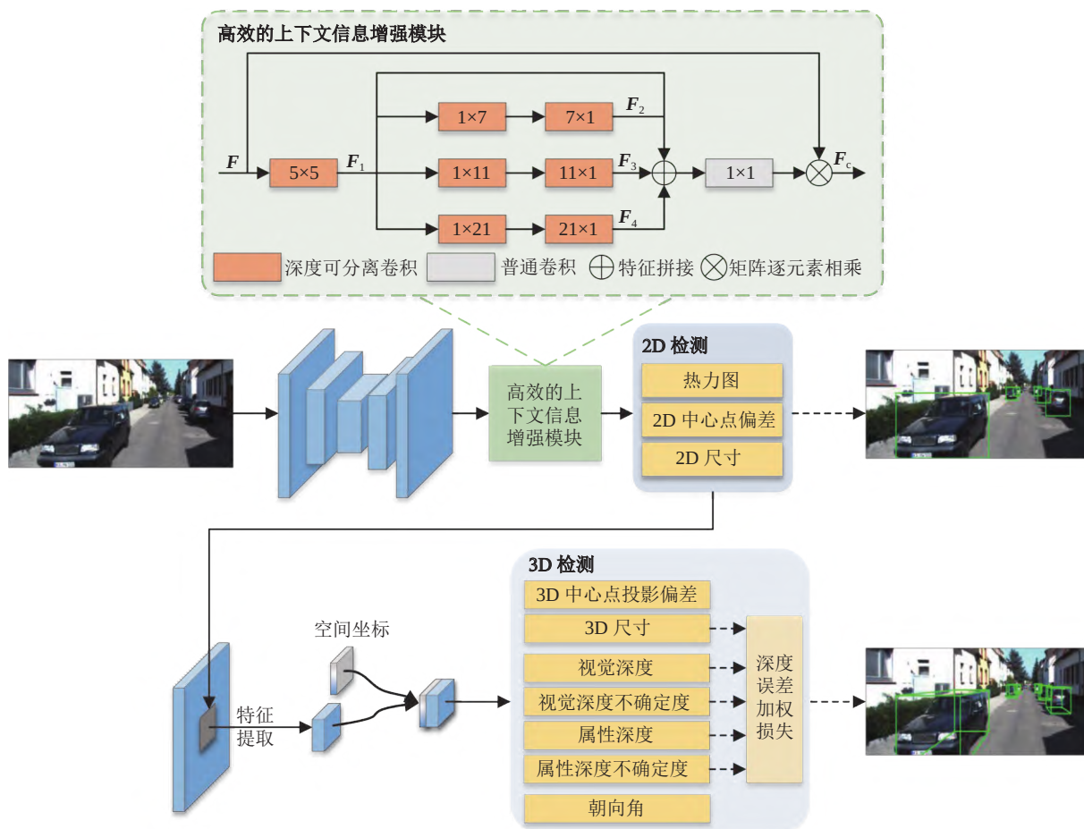
图 1 上下文信息增强和深度引导模型的架构
