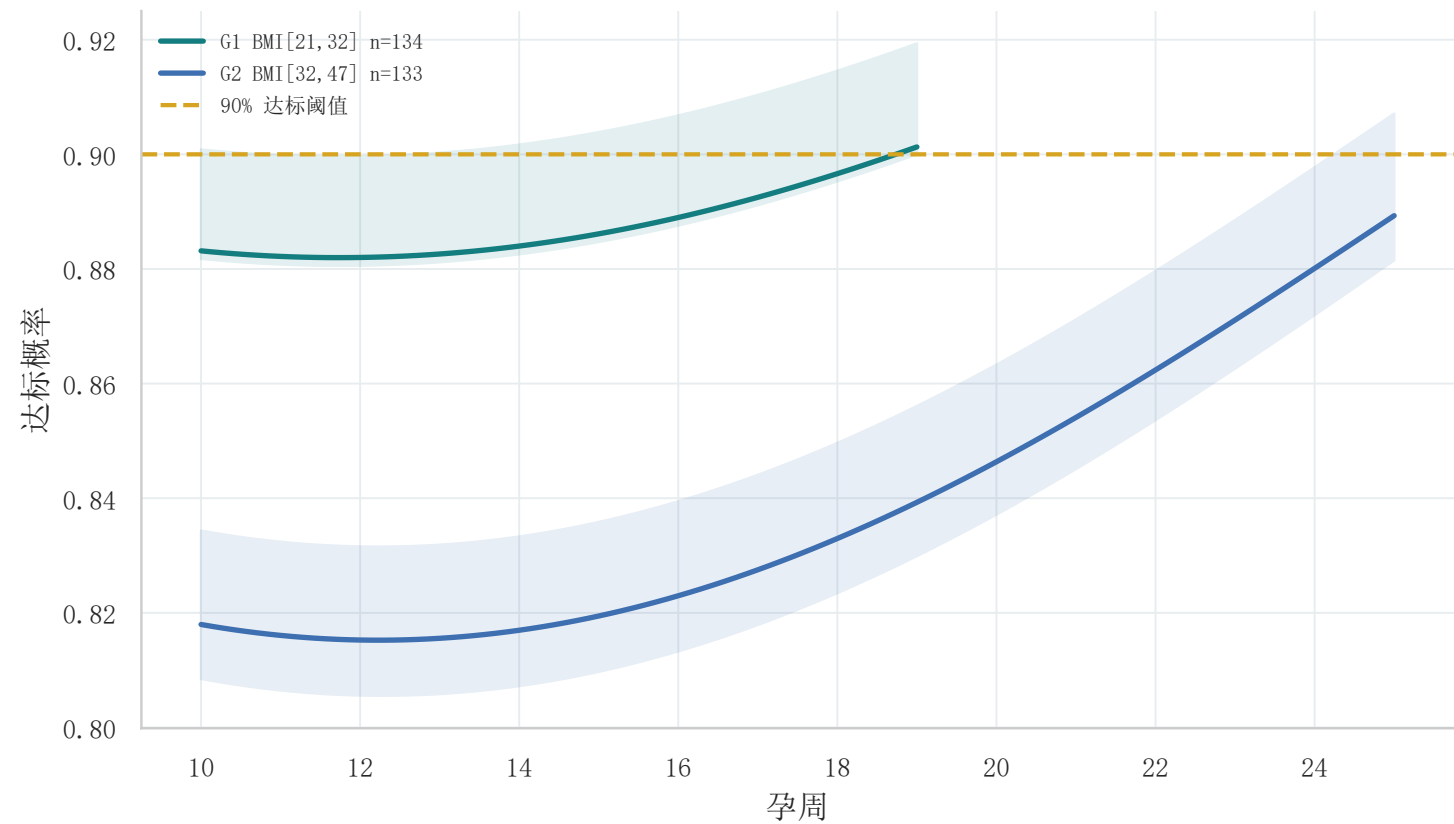
Q2 各 BMI 组达标概率曲线（区间删失 AFT）
